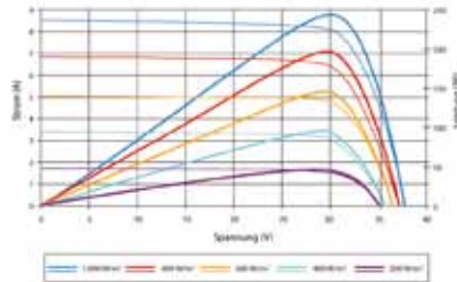
Strom-Spannungs- & Leistungs-Spannungskennlinie (245S-20)
